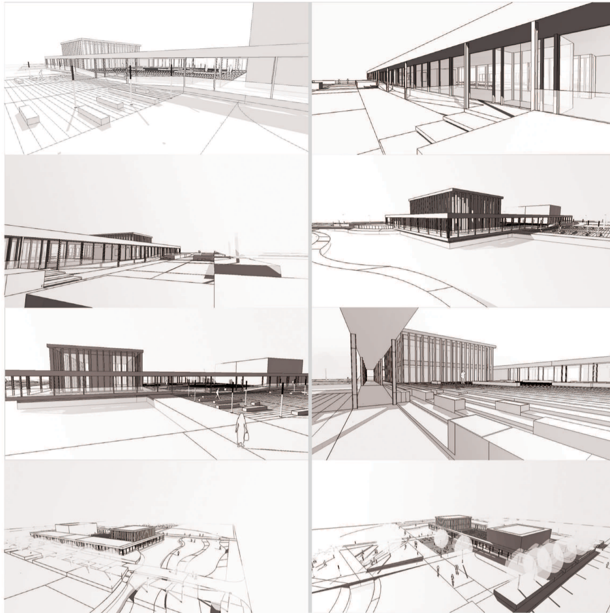
Aksonometrie - Centrum Kultury i Aktywności Lokalnej Nowe Żerniki
