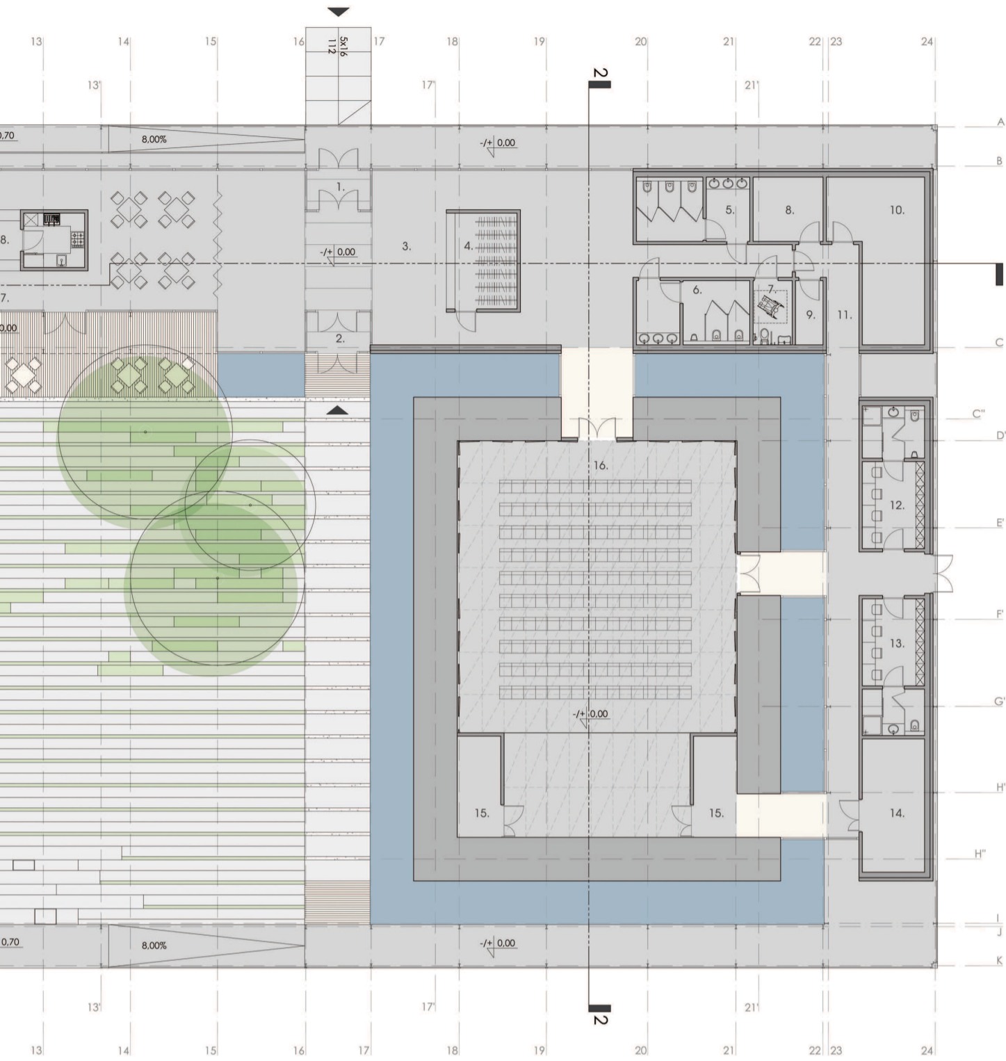
Rzut kondygnacja 0
